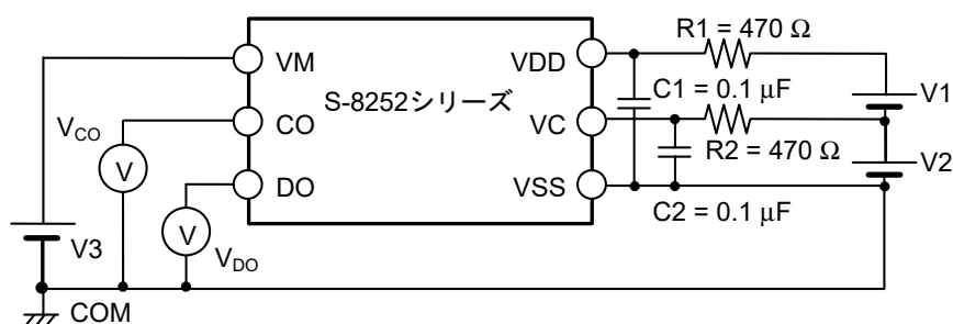
図5 測定回路1
