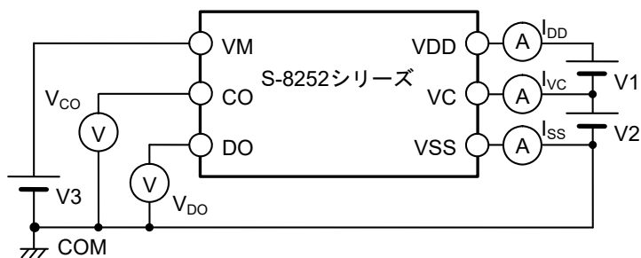
図6 測定回路2
