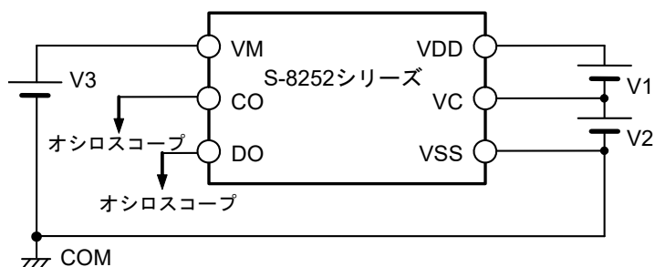
図9 測定回路5
