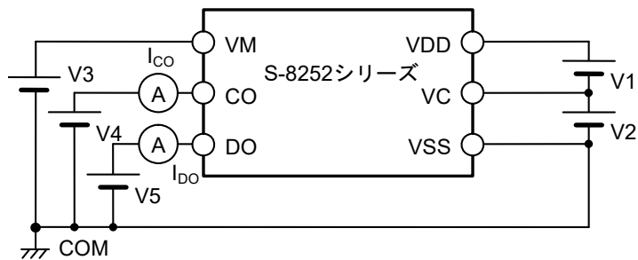
図8 測定回路4
