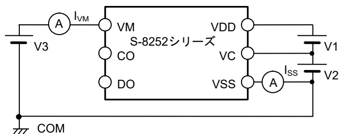
図7 測定回路3
